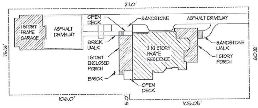
○ SITE PLAN
